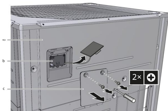
a Tấm mặt trước b PCB chính với ba màn hình 7 đoạn và ba màn hình đẩy nút c Vỏ bảo trì hộp linh kiện điện tử
