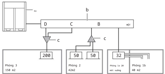
A-D Cổng ống nhánh A-D a Dàn nóng b Bộ BS c Bộ nhánh trong nhà (refnet) Phòng Phòng 32/50/200 Công suất dàn lạnh
