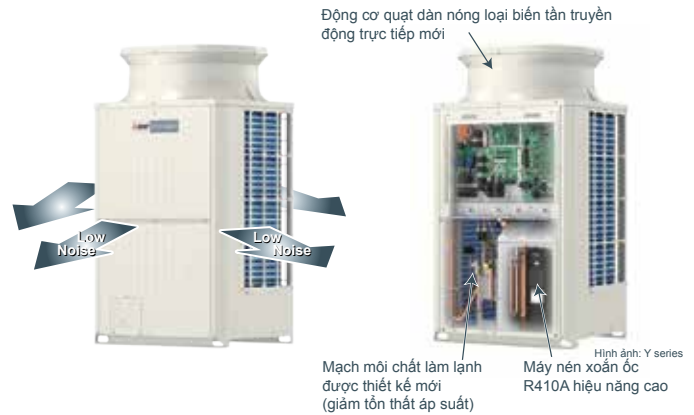
Khoang chứa máy nén được che kín để giảm độ ồn từ mọi phía.
