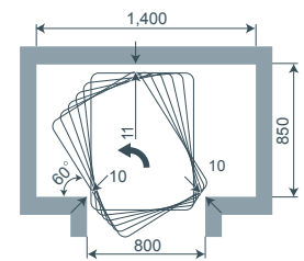
■ Ví dụ về thang máy chờ 6 người mm
