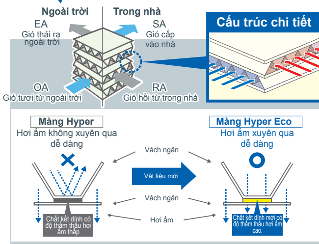
Hiệu quả trao đổi Enthalpy được cải thiện
