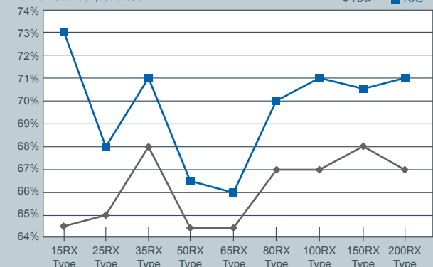
Hiệu quả trao đổi Enthalpy được cải thiện
